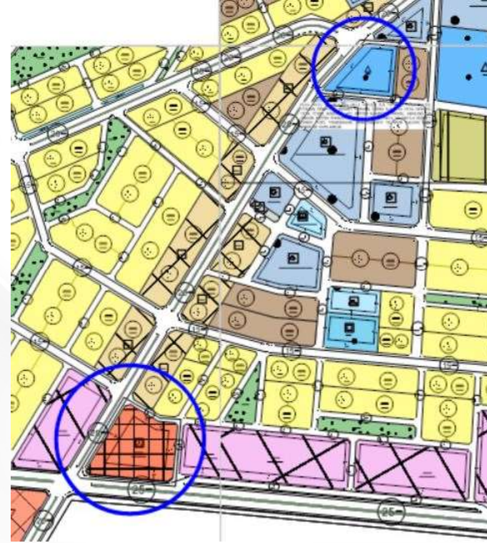
İmar Plan Değişiklik Sonrası Durum 1/1000 Uygulama İmar Planı
