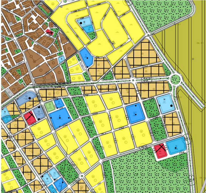
İmar Plan Değişiklik Öncesi Durum (Uzak) 1/1000 Uygulama İmar Planı
